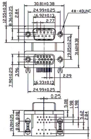
DPD-9MHD15F/Axx
